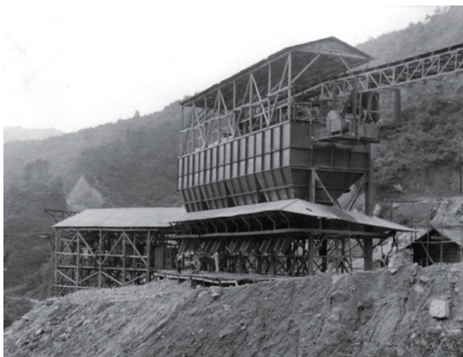
採石プラント(昭和35年頃)
